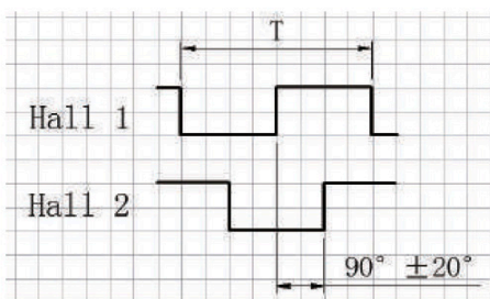
Oscillogram
